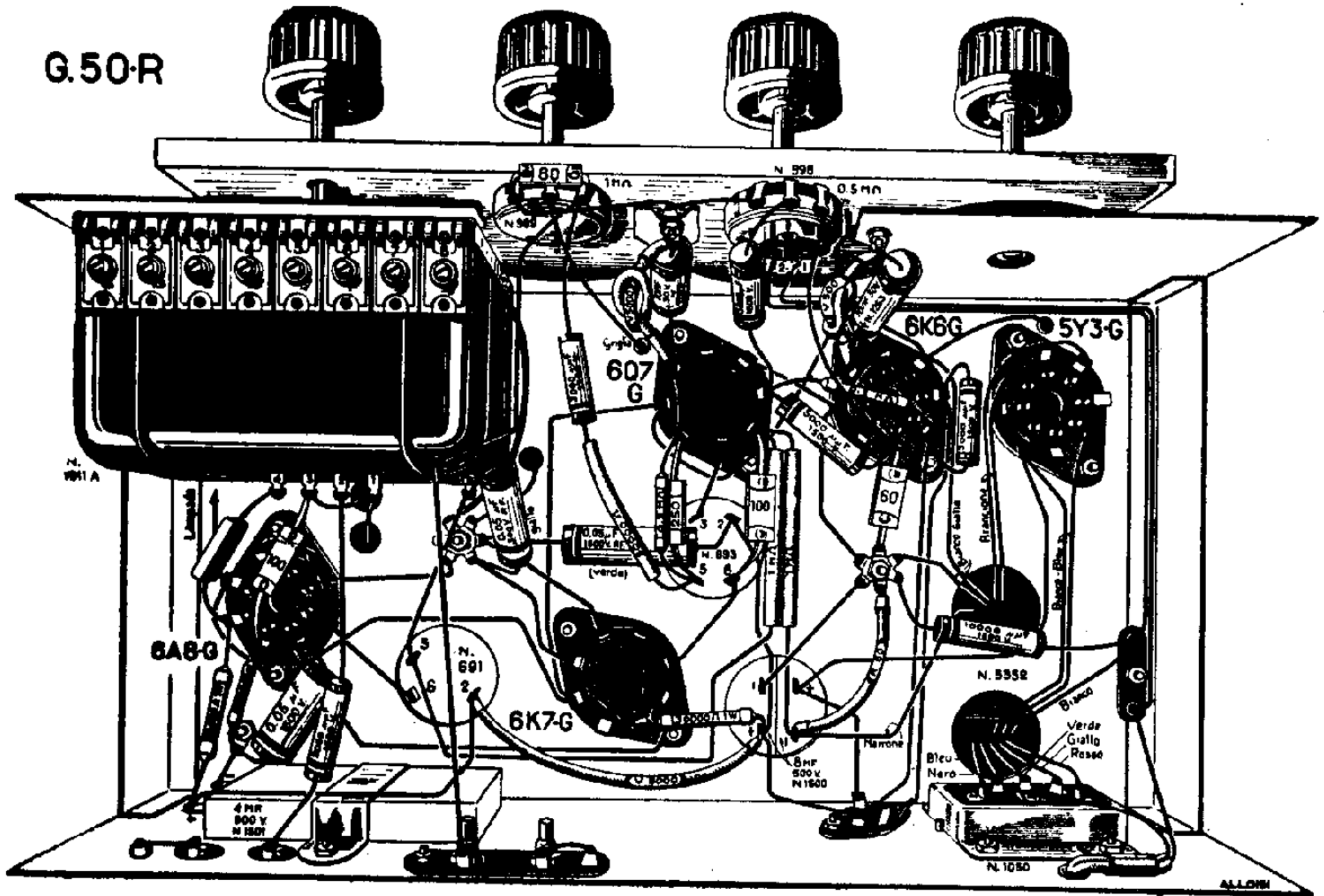
Il piano costruttivo del « G 50 R ».
